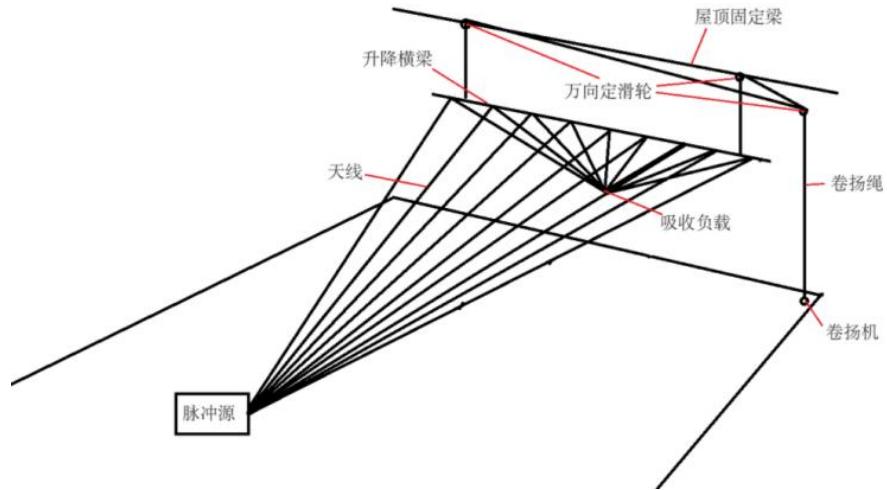
10米法暗室天线悬挂式示意图
